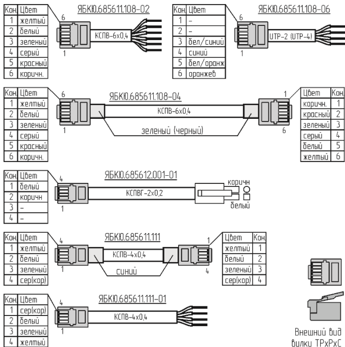
Рисунок Б.7 – Цветовая маркировка проводов кабелей
