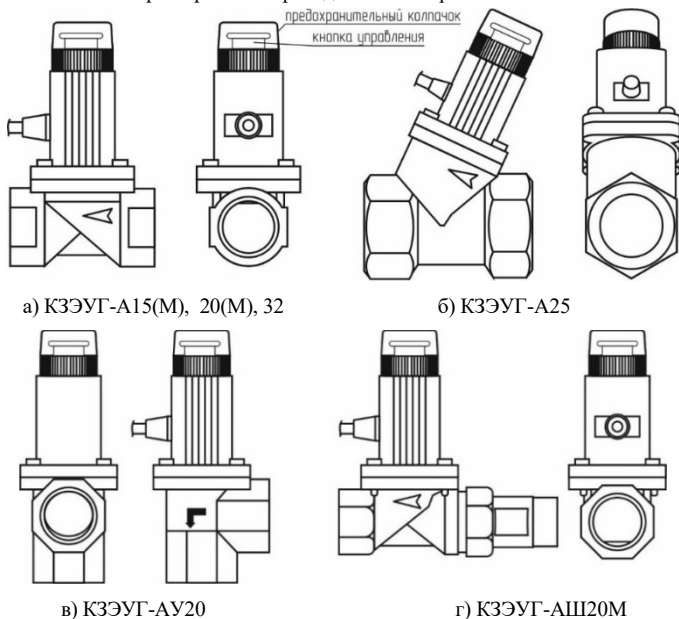
Рисунок 2 – Внешний вид клапанов КЗЭУГ-А
